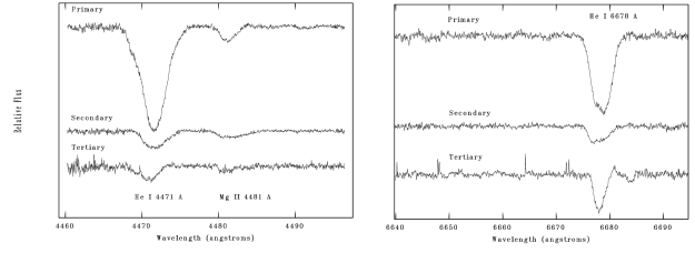
Şekil 3. Tayfinda üç bileşen barındıran CMA OB1 üyesi FM CMA'nın bileşke tayflarının farklı iki dalgaboyu bölgesinde bileşenlerine ayrıştırılması.
